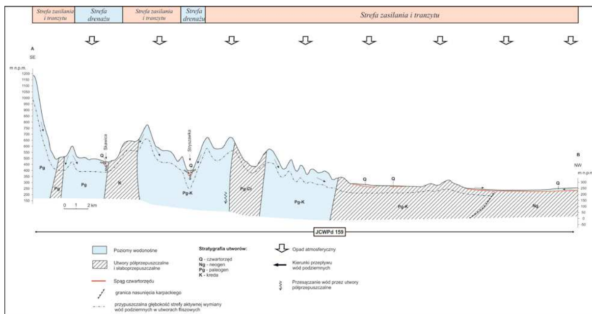
Ryc. 6. Schemat przepływu w granicach JCWPd 159.
