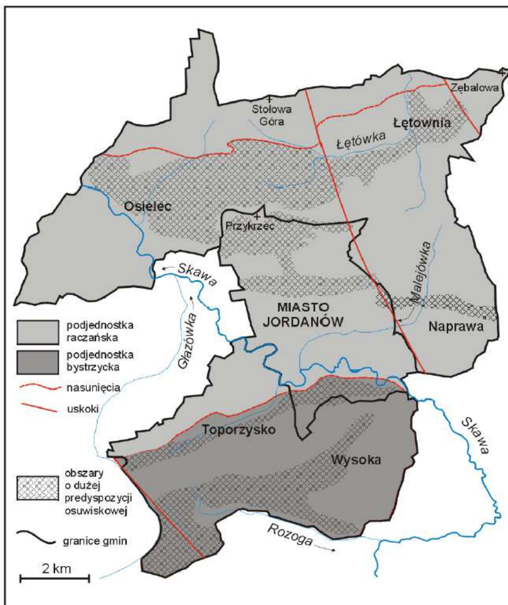
Ryc. 1. Główne jednostki strukturalne na obszarze gminy Jordanów ( Objaśnienia do mapy osuwisk i terenów zagrożonych ruchami masowymi, Gmina Jordanów, PIG, Warszawa, 2009 )
